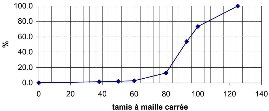
Courbe granulométrique 90/130
