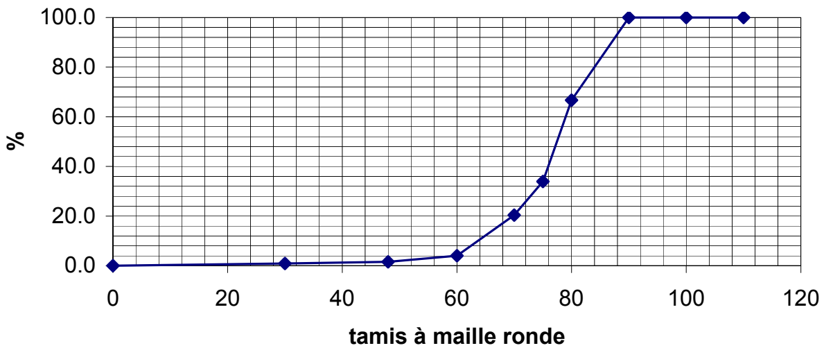
Courbe granulométrique 60/90
